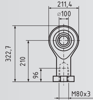
Kugelgelenkkopf GSA X K
