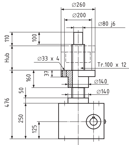
Rotierende Spindel
