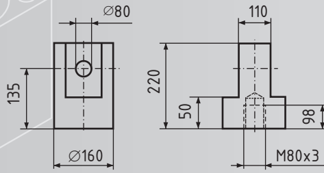
Gelenkkopf GSA X Z
