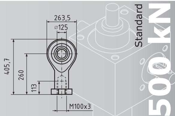
Kugelgelenkkopf GSA XI K
