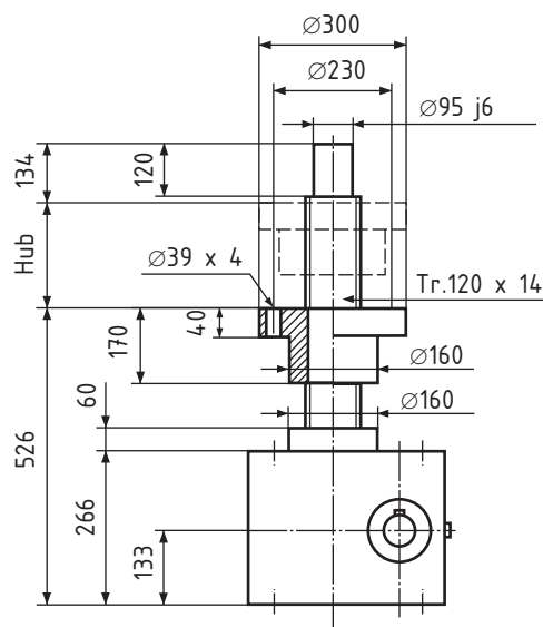
Rotierende Spindel
