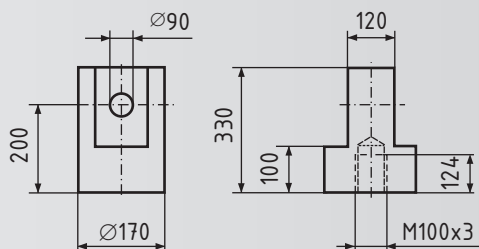
Gelenkkopf GSA XI Z
