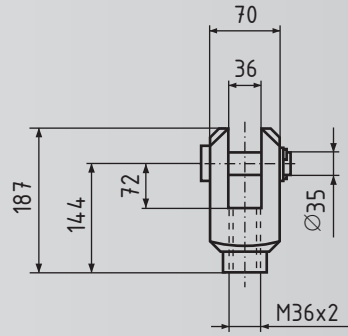
Gabelkopf GSA V G
