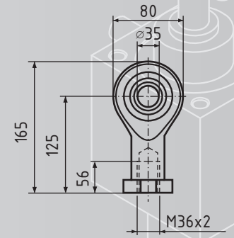
Kugelgelenkkopf GSA V K
