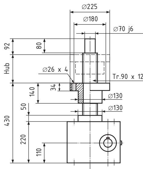
Rotierende Spindel
