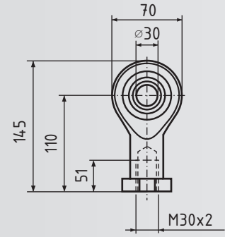
Kugelgelenkkopf GSA IV K
