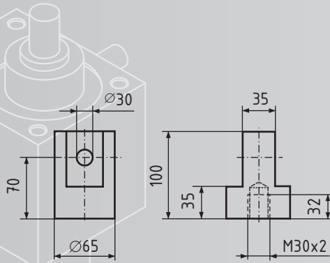
Gelenkkopf GSA IV Z
