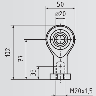
Kugelgelenkkopf GSA I K
