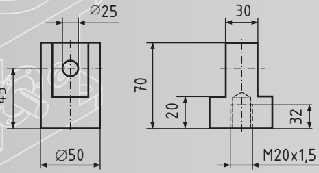
Gelenkkopf GSA IV Z S21
