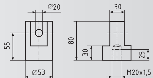
Gelenkkopf GSA III Z
