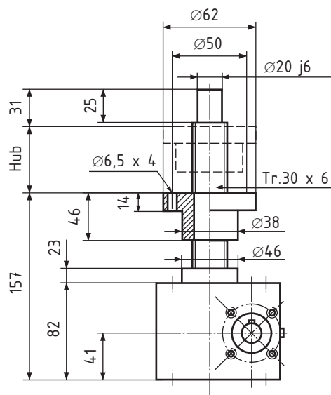
Rotierende Spindel
