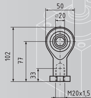
Kugelgelenkkopf GSA III K
