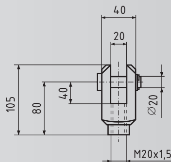
Gabelkopf GSA III G
