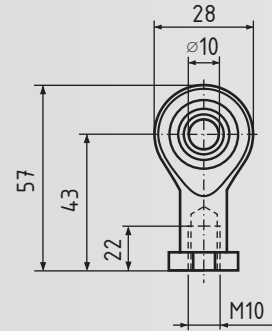
Kugelgelenkkopf GSA 0 K
