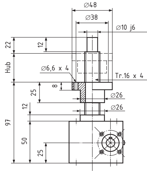
Rotierende Spindel
