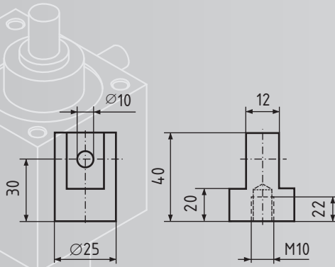
Gelenkkopf GSA 0 Z
