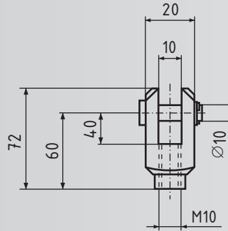
Gabelkopf GSA 0 G
